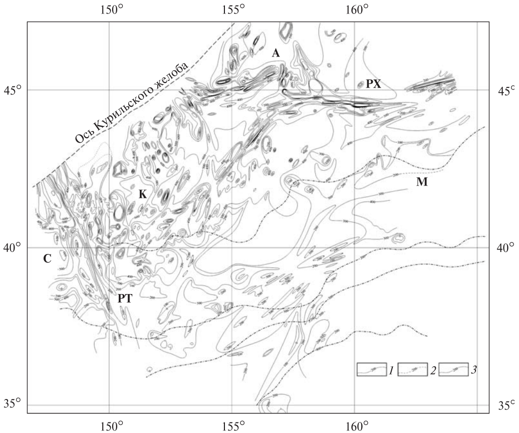
Рис. 2. Карта изопакит осадочного кайнозоя (1 — установленные, 2 — предполагаемые) и над-базальтового позднего мезозоя (3). Изопакиты в метрах [2]. А, К, С — фаны Авачинского, среднекурильских и Сангарского каньонов; М — Камчатский контурный мегафан; РХ, РТ — разломы Хоккайдо и Тускарора
