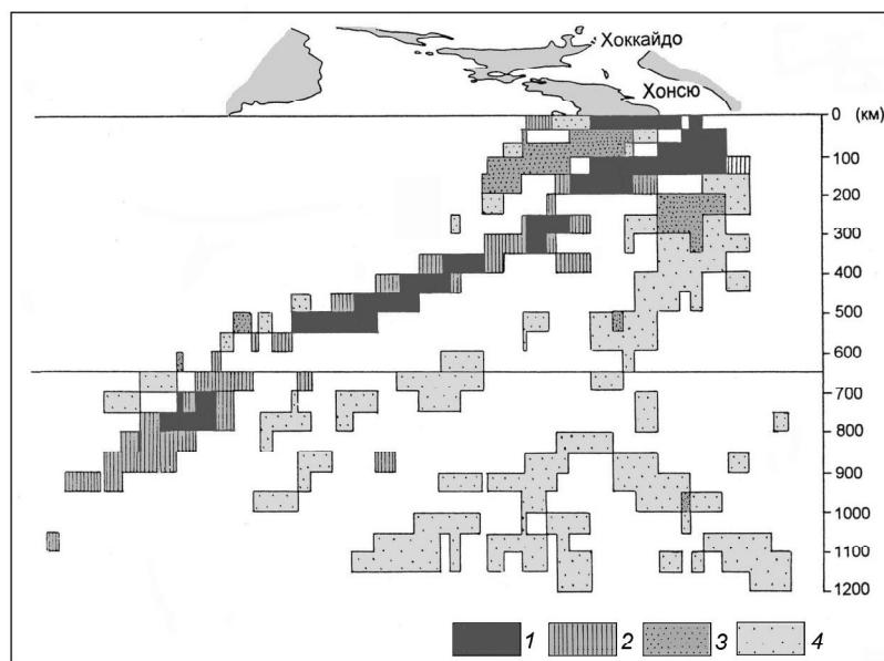
Рис. 2. Томографический скоростной разрез на основе Р-волн по профилю: район Владивостока – северная часть о-ва Хонсю [31].
