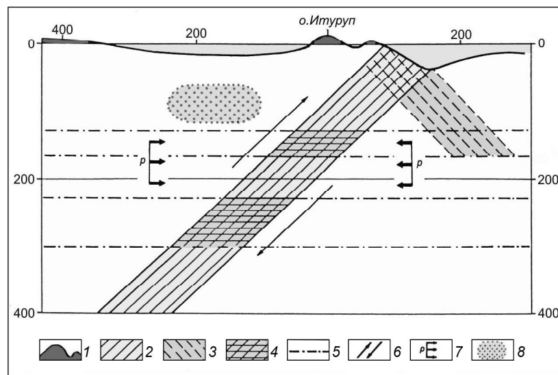
Рис. 1. Схема образования сейсмофокальной зоны как системы глубинных нарушений под влиянием постоянно действующих горизонтальных сил сжатия на границе континентальных и океанических структур [20, 32].
