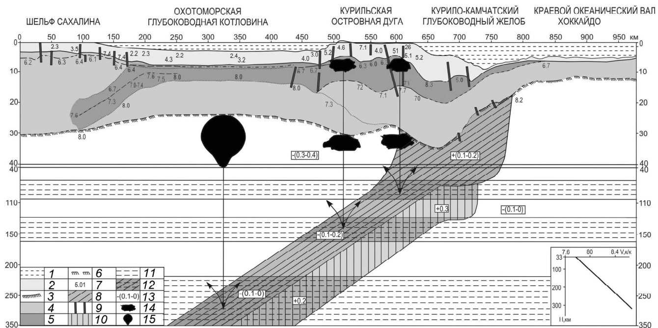
Рис. 4. Сводный график, отражающий строение земной коры зоны перехода от континента к океану [17] и зоны магмообразования Курильской сейсмофокальной зоны [22].
