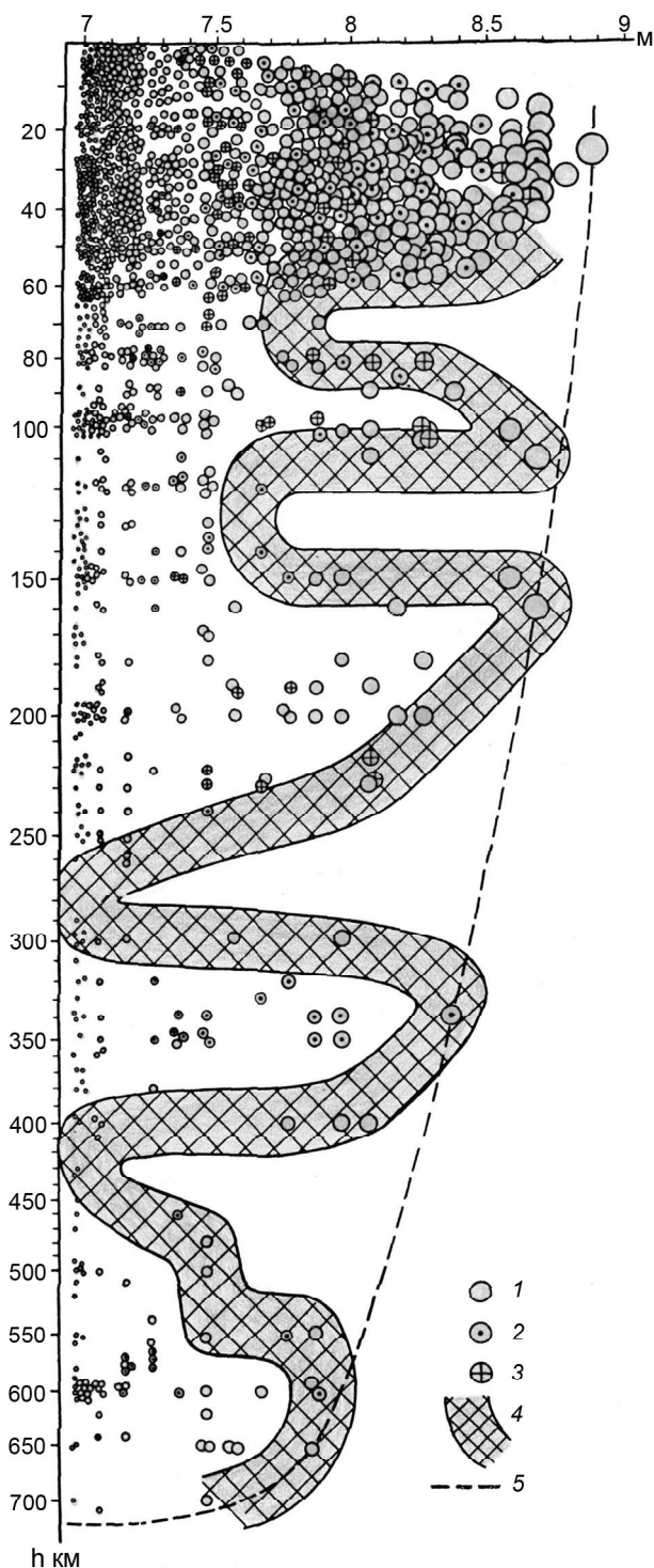
Рис. 3. Полиастеносферная модель строения верхней мантии ( M_{\max} = f(h) ), отражающая изменение прочностных свойств среды с глубиной h [23].
