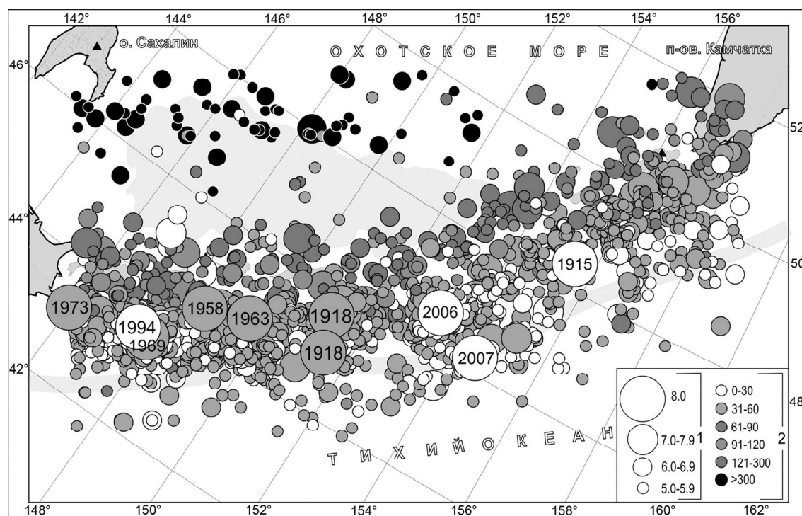
Рис. 5. Карта эпицентров землетрясений с M \geq 5 Курило-Камчатского региона (1737–2009 гг.) с классификацией землетрясений по магнитуде (1) и глубине очага (2) [8].
